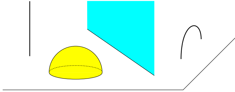
FIGURE 7. Rette e piani in \mathbb{H}^3 visualizzate con il modello del semispazio.
