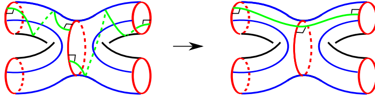
FIGURE 13. Una torsione di un opportuno angolo \theta permette di far combaciare le curve verdi minimizzando le intersezioni con le curve blu.
