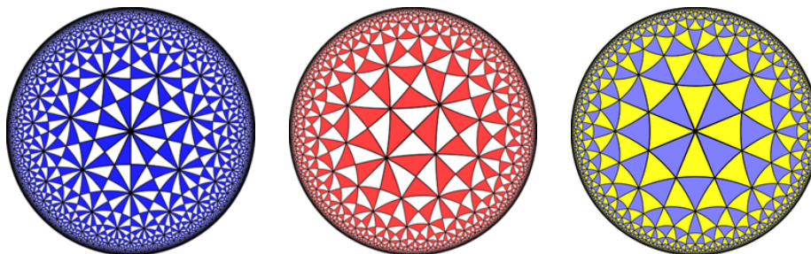
FIGURE 7. Le tassellazioni (2, 3, 7) , (2, 4, 5) e (3, 3, 4) nel piano iperbolico.
