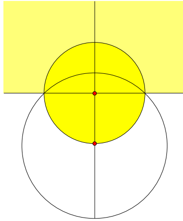
FIGURE 6. L'inversione lungo la sfera di centro (0, \dots, 0, -1) e raggio \sqrt{2} trasforma il disco di Poincaré nel semispazio.
