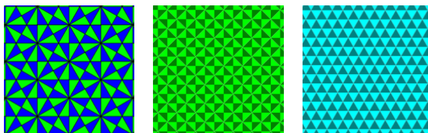
FIGURE 6. Le tassellazioni (2, 3, 6) , (2, 4, 4) e (3, 3, 3) nel piano.
